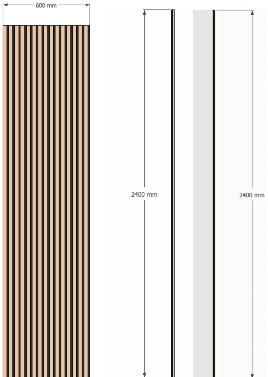
Vues latérales
